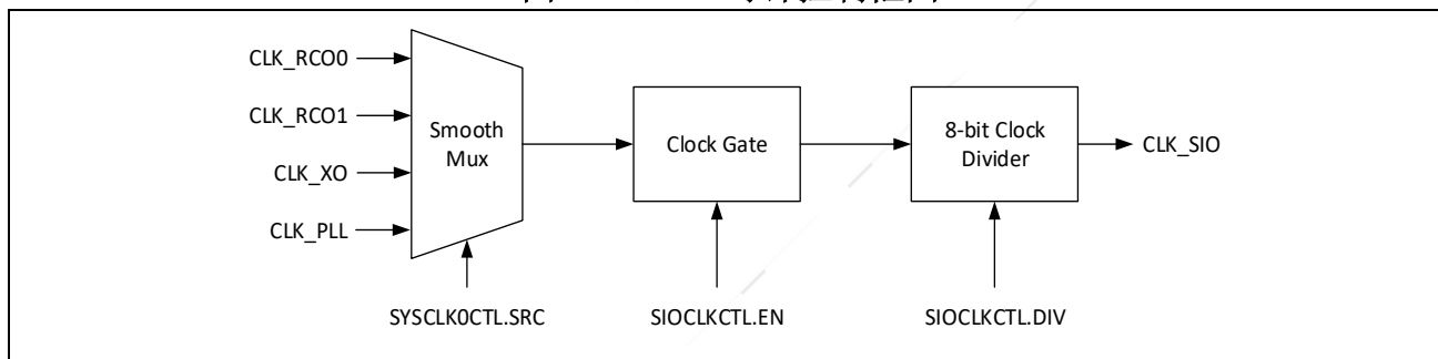
图 3-16: SIO 时钟控制框图
