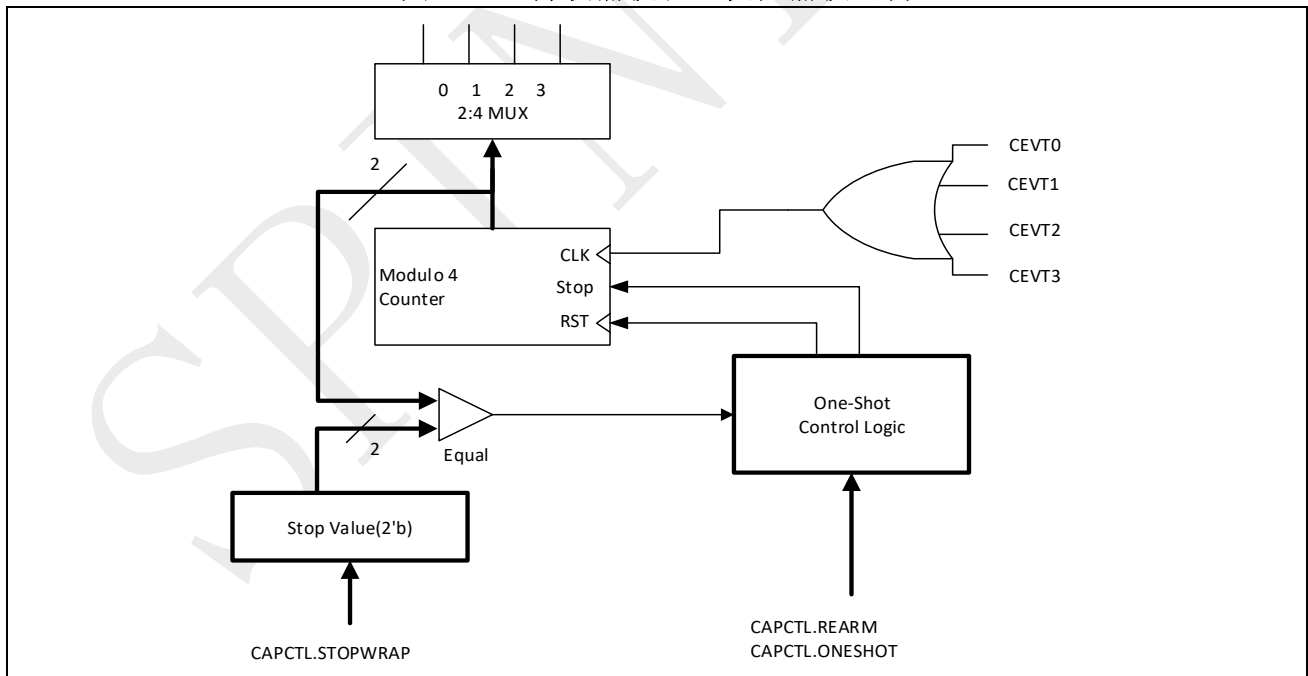
图 11-6：持续捕获和一次性捕获逻辑
