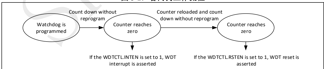
图 9-1：看门狗工作流程
