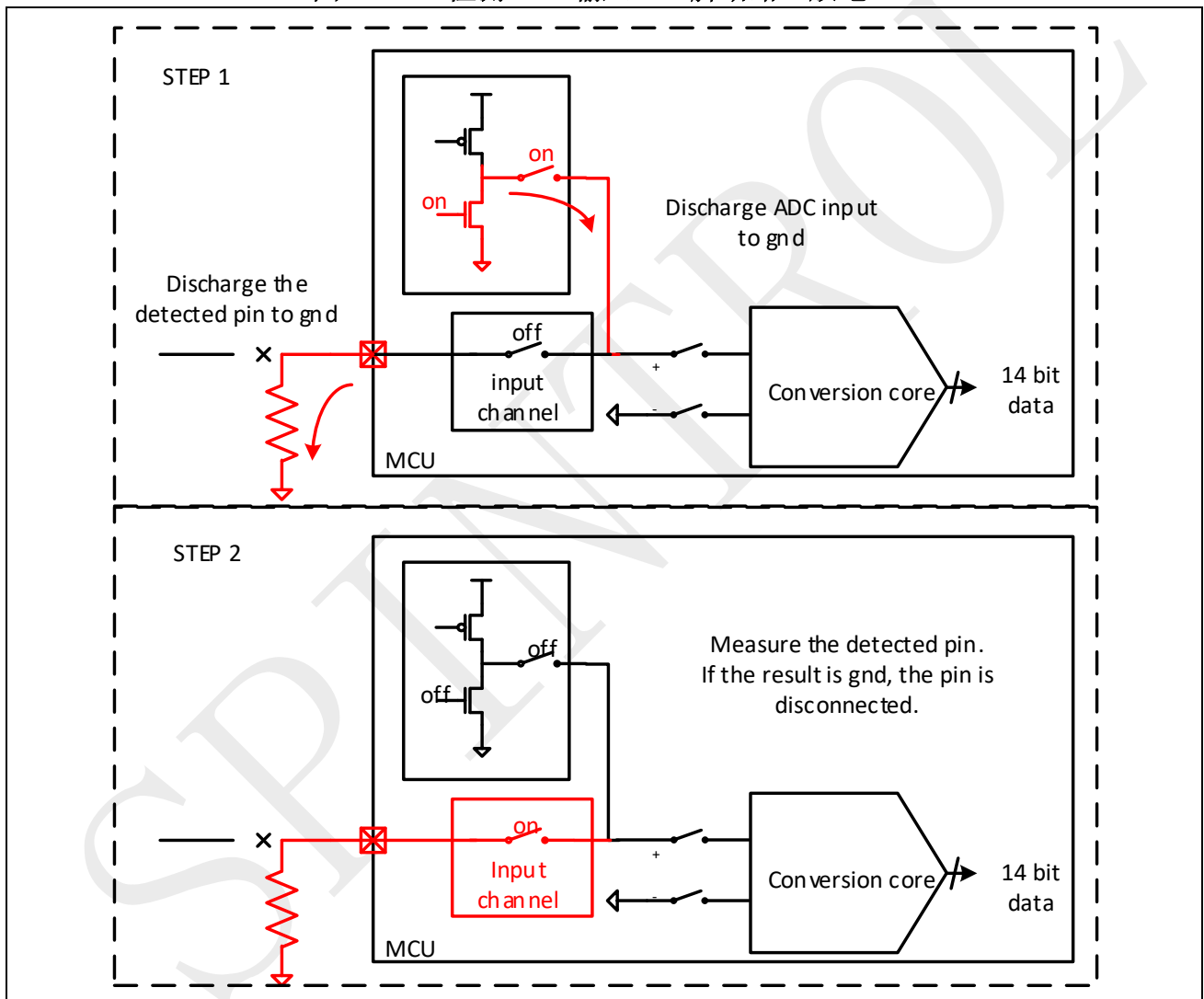
图 12-16: 检测 ADC 输入 PIN 脚断路（放电）
