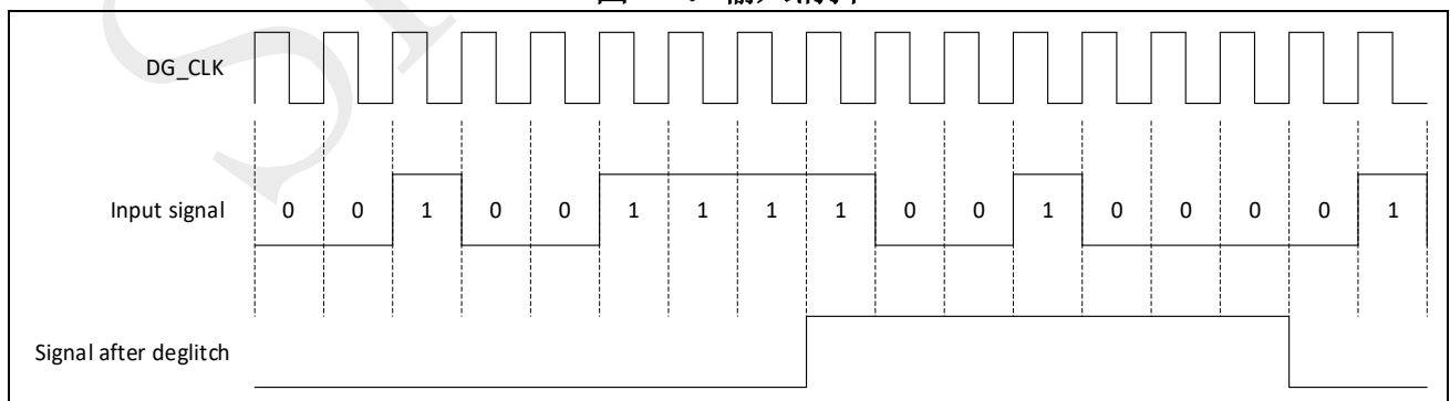
图 4-4：输入消抖
