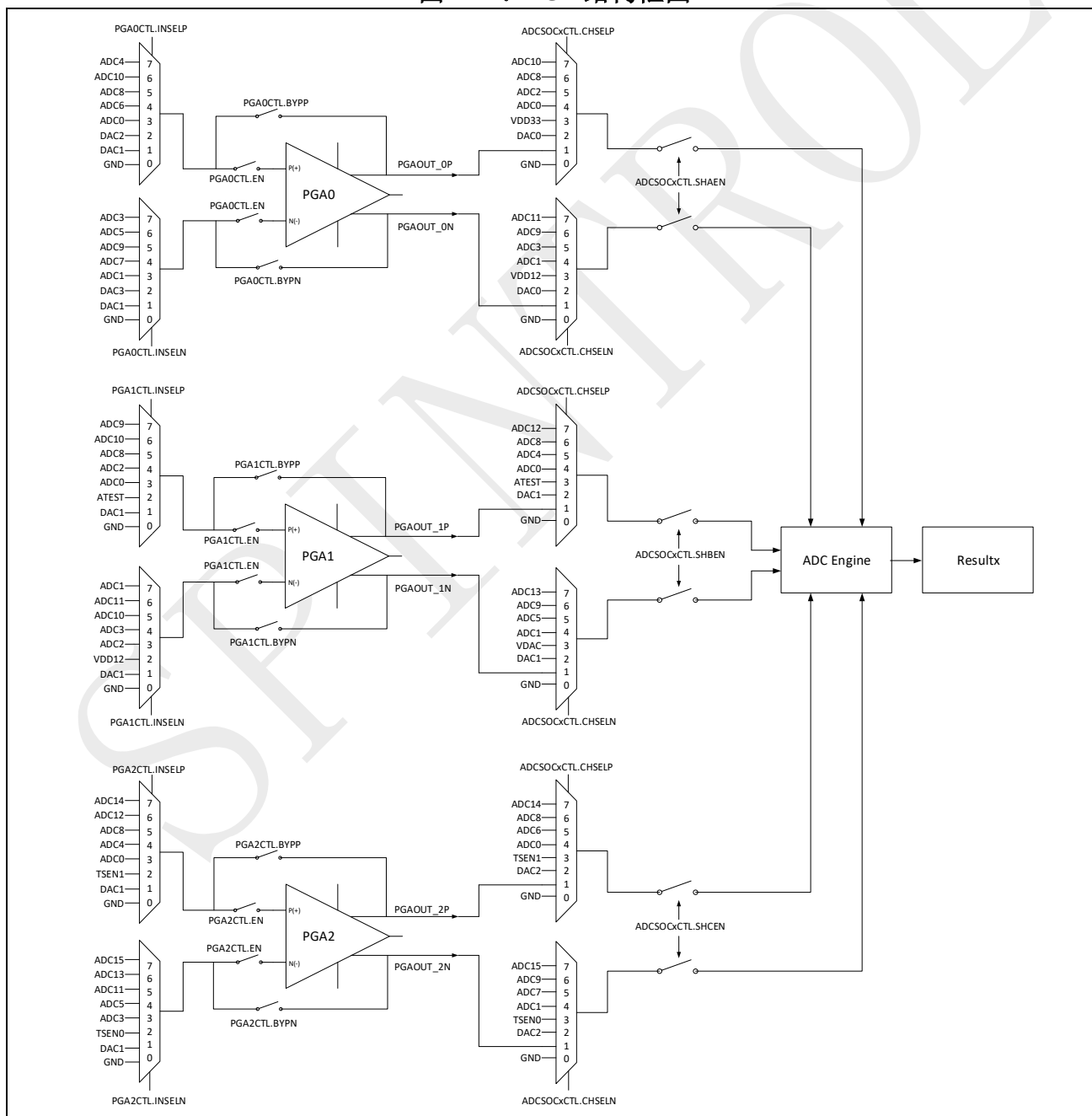
图 14-1: PGA 结构框图
