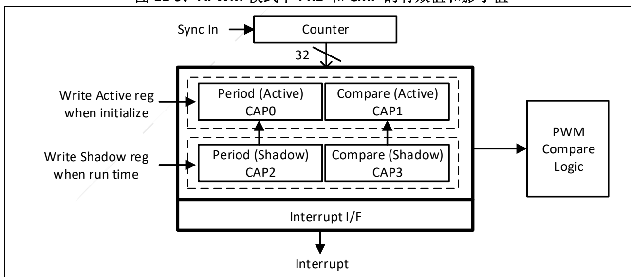
图 11-9: APWM 模式下 PRD 和 CMP 的有效值和影子值
