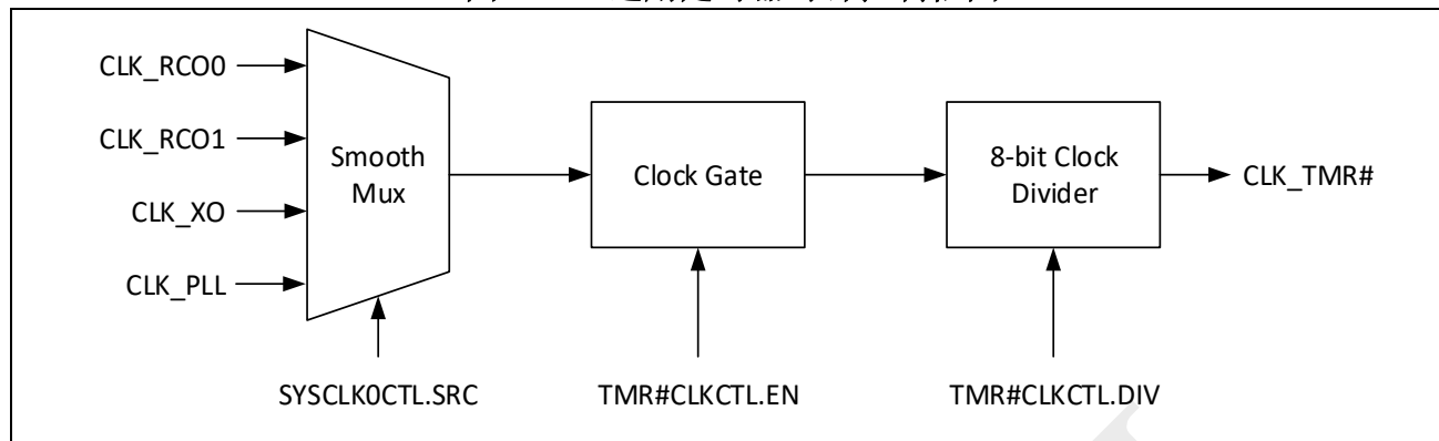
图 3-12: 通用定时器时钟控制框图
