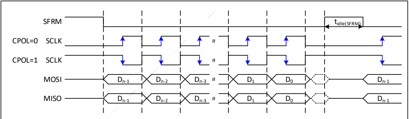
图 21-4: CPHA=1 时序图
