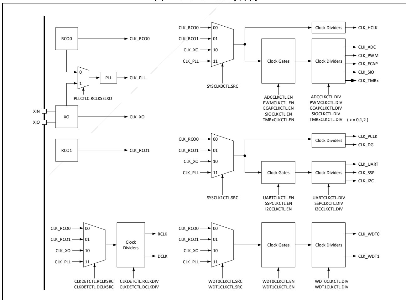
图 1-2: SPC1168 时钟树
