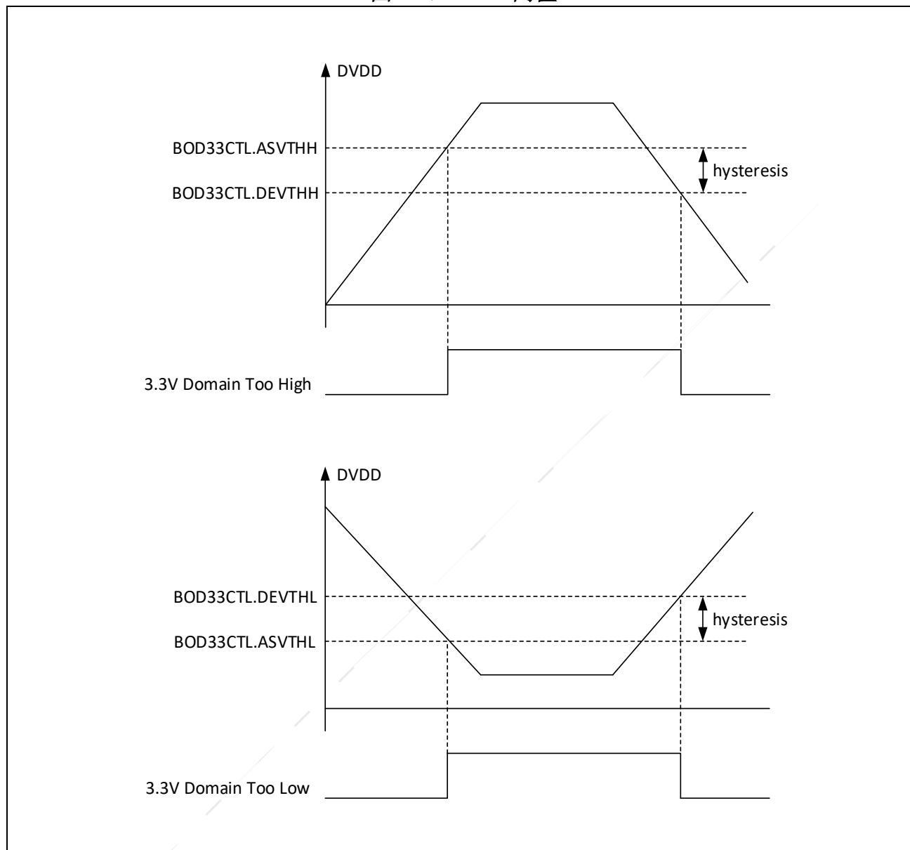
图 2-4: DVDD 阈值
