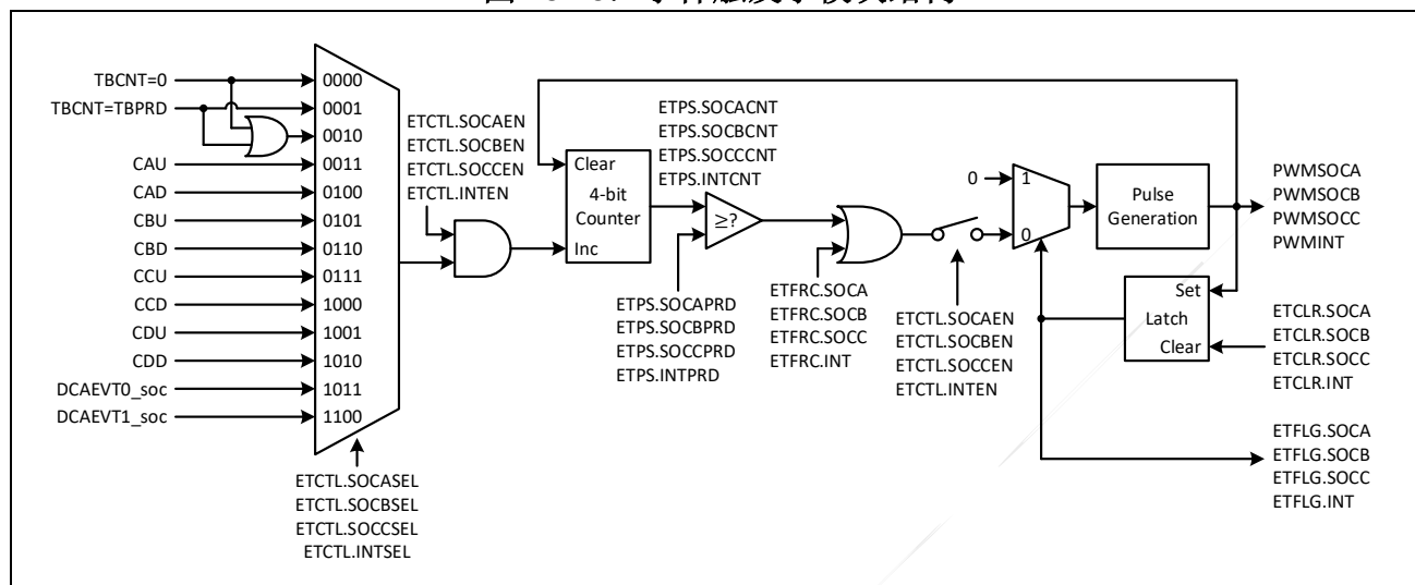
图 10-20：事件触发子模块结构
