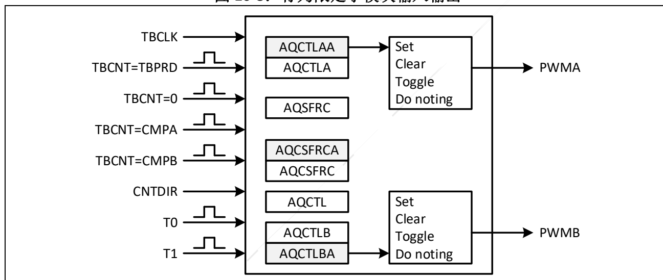
图 10-8：行为限定子模块输入输出
