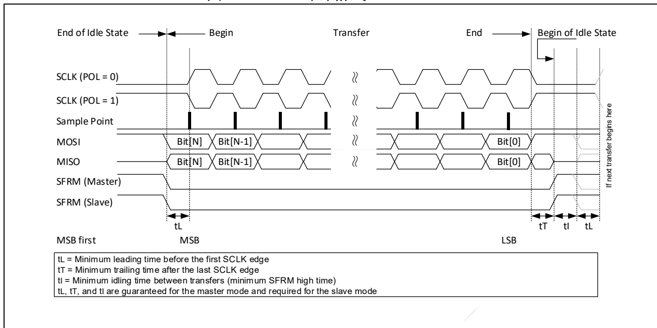
图 19-4: SSP 时钟格式 0 (PHS = 0)
