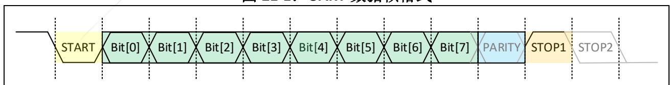
图 21-1: UART 数据帧格式
