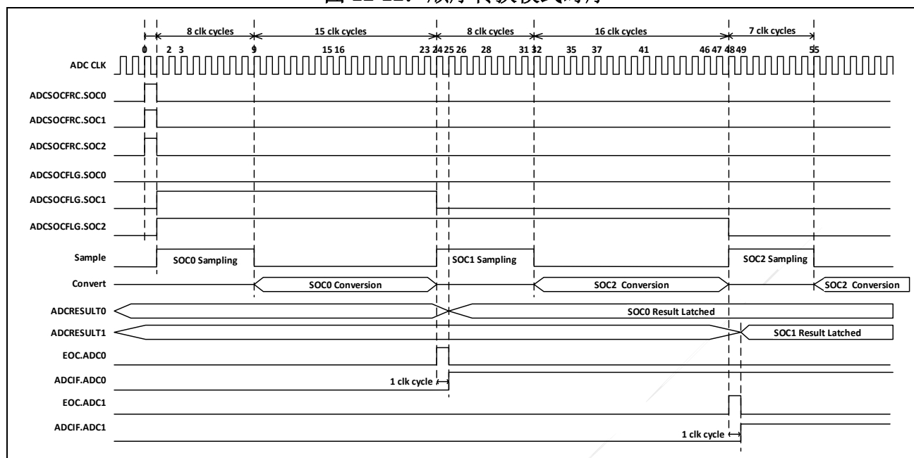
图 12-13: 同时采样模式时序
