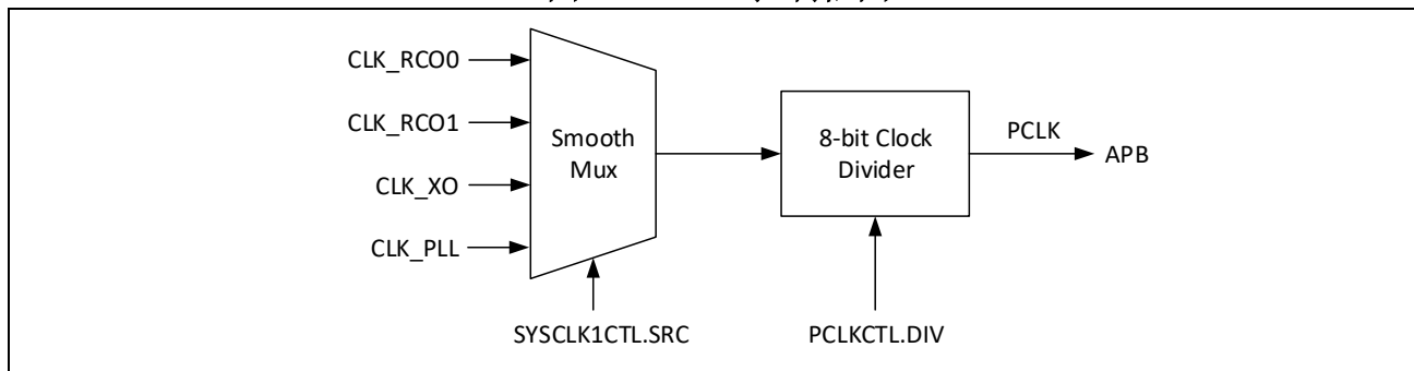
图 3-8: PCLK 控制框图
