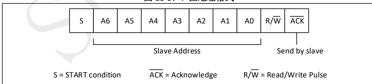
图 18-3: 7 位地址格式
