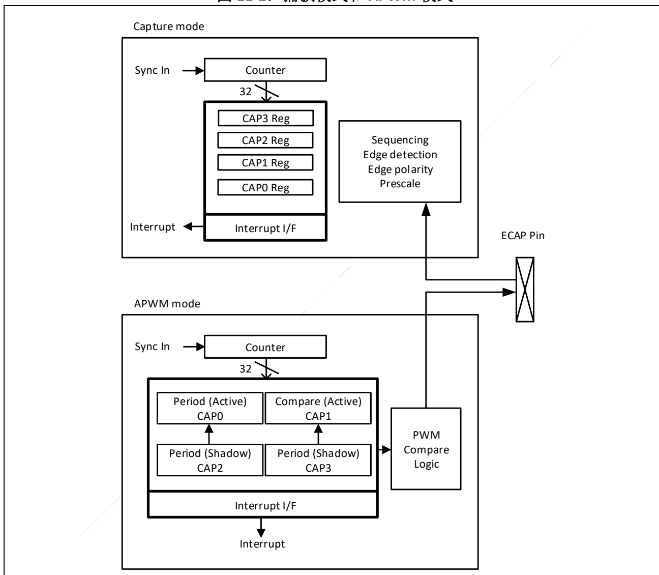
图 11-2: 捕获模式和 APWM 模式
