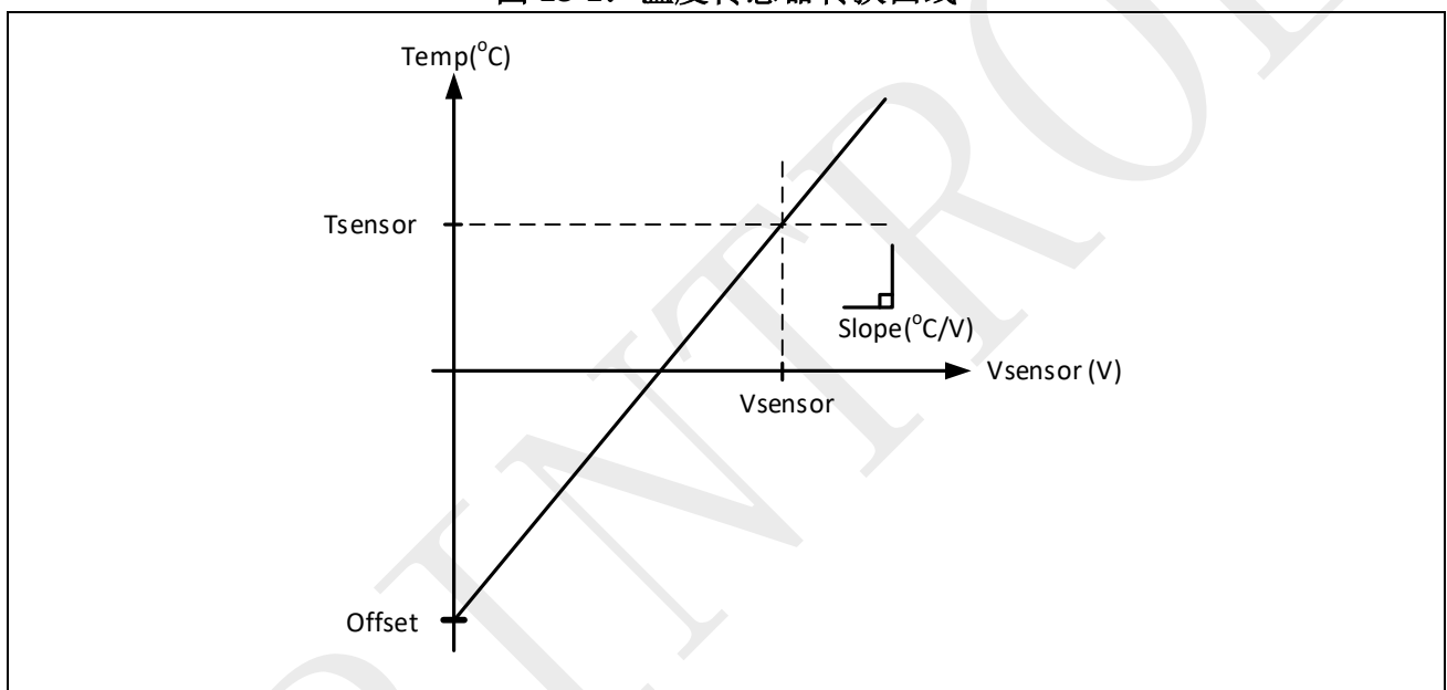
图 13-1：温度传感器转换曲线
