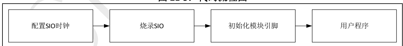
图 21-5：代码流程图
