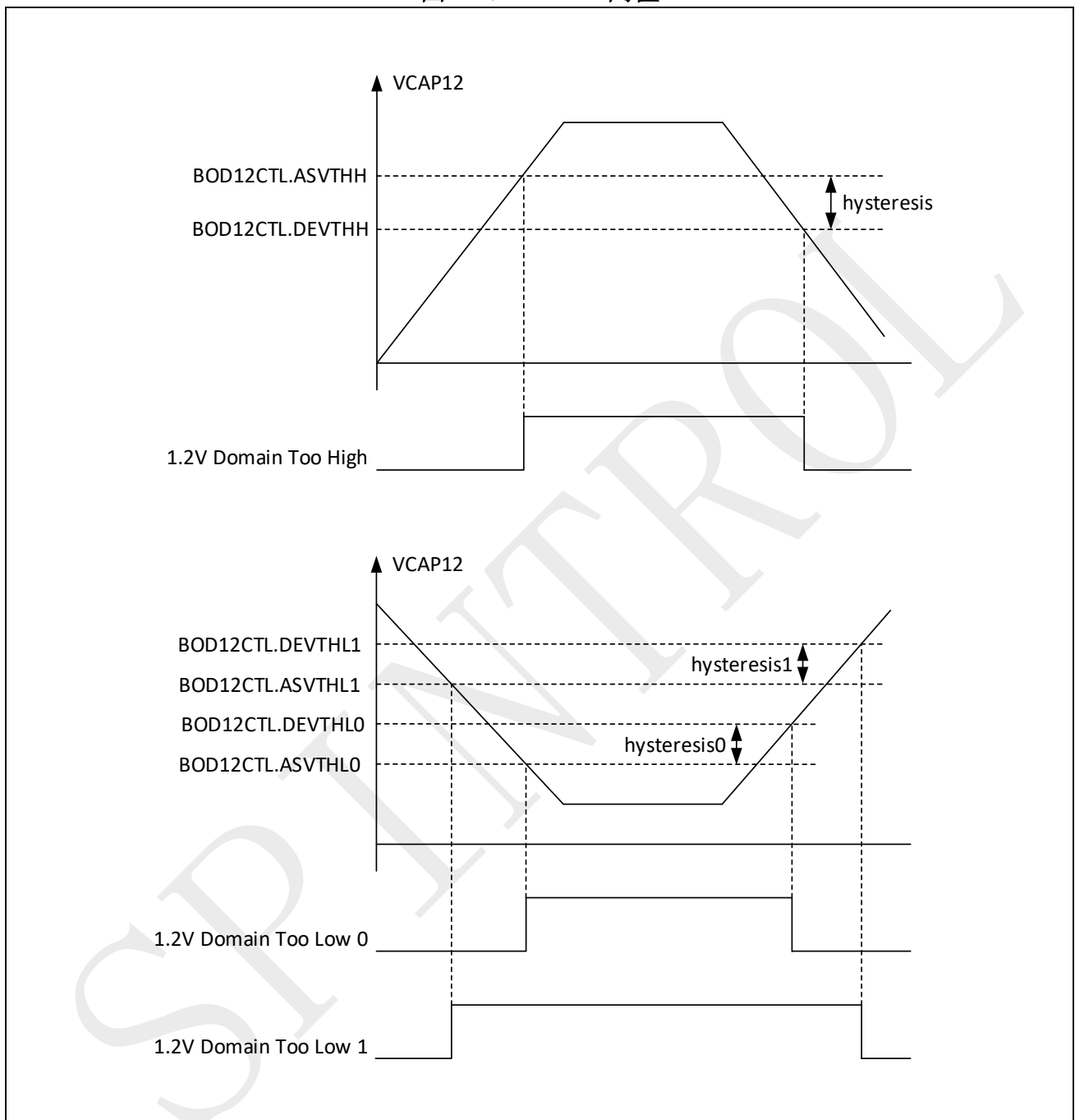
图 2-5: VCAP12 阈值
